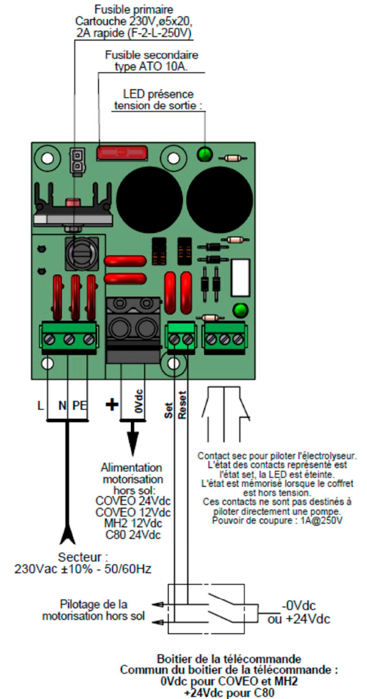
C80 (Coffret 24V)
